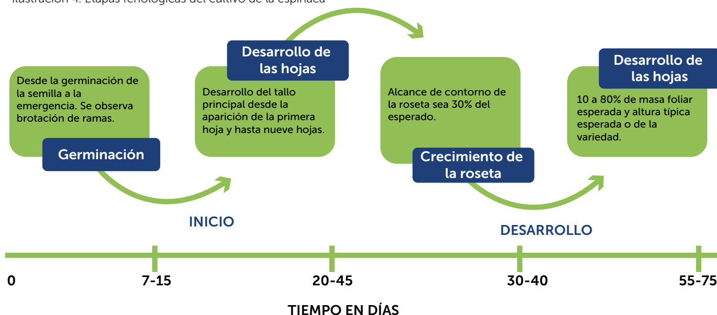
Ilustración 4. Etapas fenológicas del cultivo de la espinaca
